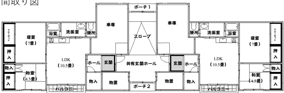
間取り図
