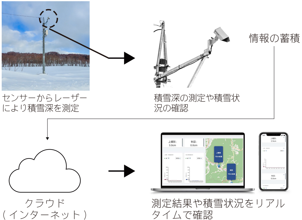
図 1 除雪モニター実証実験のイメージ
